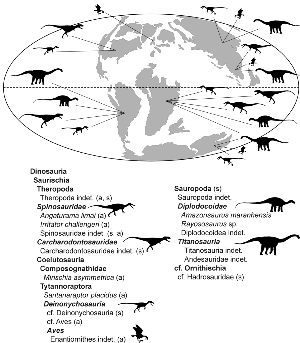
Figura 2 Reconstituição paleogeográfica do Cretáceo Inferior (~ 100 Ma), modificado de Blakey (2006). As silhuetas no mapa indicam a ocorrência em outras áreas dos principais grupos de dinossauros registrados no Brasil durante o Aptiano-Cenomaniano, mostrados na lista. (a): espécimes provenientes da Formação Santana, Bacia do Araripe; (s): Bacia de São Luís-Grajaú. As silhuetas referem-se aos grupos encontrados no Brasil, colocadas à frente dos nomes sublinhados, aos quais correspondem. Fonte: Weishampel et alii (2004); Curry-Rogers (2005); Machado & Kellner (2005); Makovicky et alii (2005).
