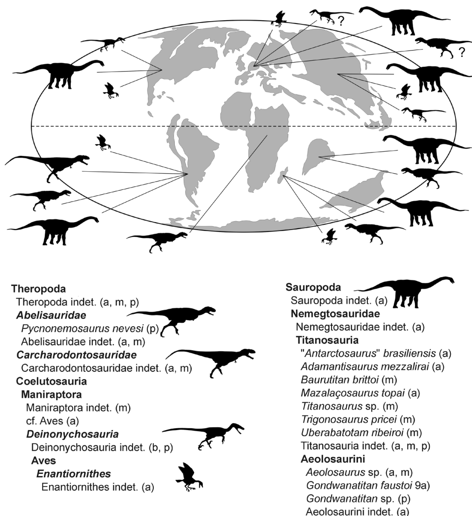
Figura 3 Reconstituição paleogeográfica do Cretáceo Superior (~ 65 Ma), modificado de Blakey (2006). As silhuetas no mapa indicam a ocorrência em outras áreas dos principais grupos de dinossauros registrados no Brasil durante o Campaniano-Maastrichtiano, mostrados na lista. (a): espécimes provenientes da Formação Adamantina; (m): Formação Marília; (b): Grupo Bauru; (p): Grupo Parecis. As silhuetas referem-se aos grupos encontrados no Brasil, colocadas à frente dos nomes sublinhados, aos quais correspondem. Fonte: Weishampel et alii (2004); Smith & Lamanna (2006); Krause et alii (2007).
