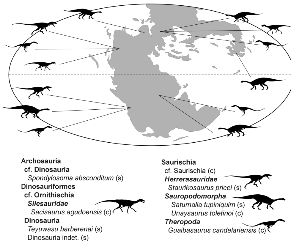
Figura 1 Reconstituição paleogeográfica do Triássico Superior (~ 220 Ma), modificado de Blakey (2006). As silhuetas no mapa indicam a ocorrência em outras áreas dos principais grupos de dinossauros registrados no Brasil durante o Carniano-Noriano, mostrados na lista. (s): espécimes provenientes da Formação Santa Maria; (c): espécimes provenientes da Formação Caturrita. As silhuetas referem-se aos grupos encontrados no Brasil, colocadas à frente dos nomes sublinhados, aos quais correspondem. Fonte: Langer et alii (2010).
